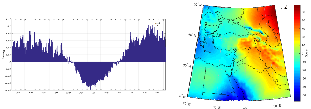
شکل ۵: الگوی مکانی نمرات مؤلفه دوم فشار تراز دریا (الف) و توزیع زمانی بردار ویژه مؤلفه دوم فشار تراز دریا (ب)
