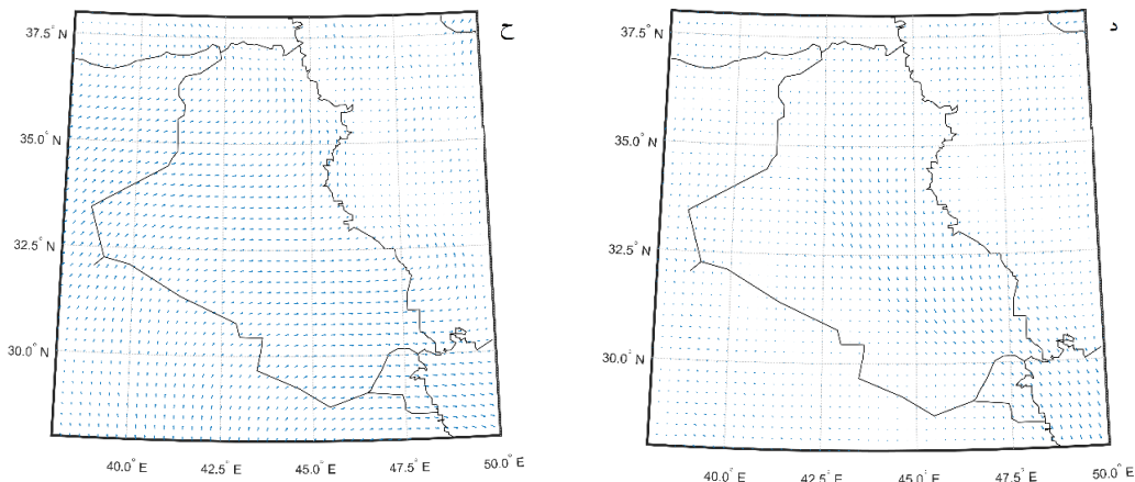
شکل ۱۱: جهت وزش باد در تراز ۱۰۰۰، (الف) زمستان، (ب) بهار، (ج) تابستان، (د) پاییز و جهت وزش باد در تراز ۸۵۰، (ه) زمستان، (و) بهار، (ز) تابستان، (ح) پاییز تهیه و ترسیم: نگارندگان، ۱۴۰۳
