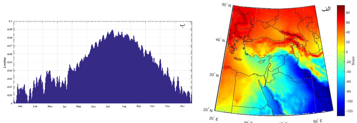
شکل ۴: الگوی مکانی نمرات مؤلفه اول فشار تراز دریا (الف) و توزیع زمانی بردار ویژه مؤلفه اول فشار تراز دریا (ب)
