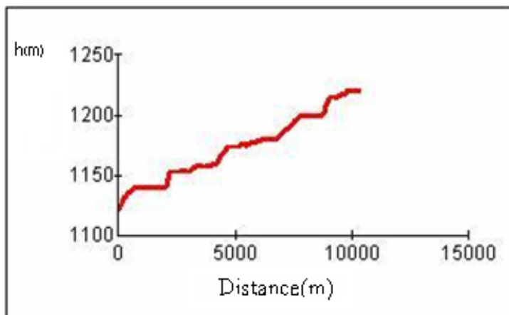
شکل ۱۰: نیمرخ طولی رودخانه چله شماره ۳ مأخذ: نقشه توپوگرافی ۱:۵۰۰۰۰ کال کش و محاسبات نگارنده
