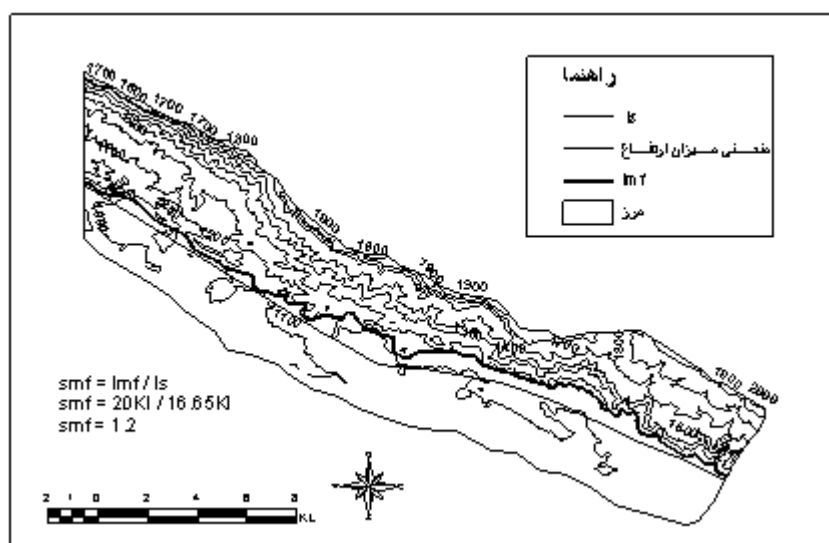
شکل ۵: محاسبه‌ی شاخص سینوسی جبهه‌ی کوهستان مأخذ: نقشه‌ی توپوگرافی ۱:۵۰۰۰۰ کال کش و محاسبات نگارنده
