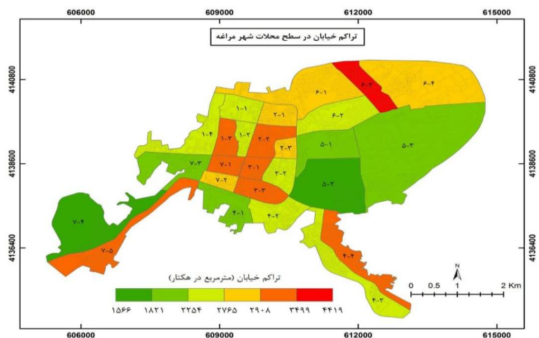
شکل ۵: تراکم خیابان در سطح محلات شهر مراغه
