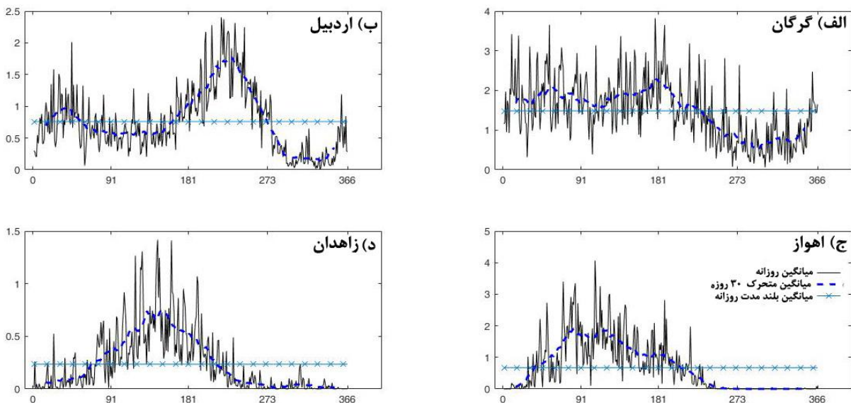
شکل ۲: میانگین مجموع بارش روزانه، میانگین بلندمدت روزانه (۳۶۶ روزه) و میانگین متحرک ۳۰ روزه بارش چهار ایستگاه منتخب
