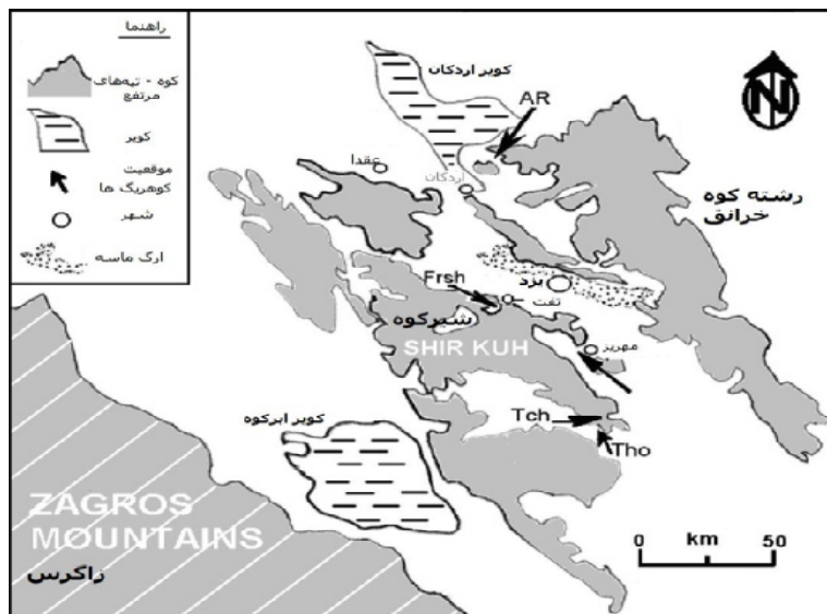
شکل ۲: موقعیت کوهریگ‌های مهم در استان یزد (محل کوهریگ‌ها با پیکان مشخص شده است). حروف اختصاری: AR اردکان، Frsh فراشاه تفت، Tch تنگ چنار، Tho تنگ حوضکی. مأخذ: نگارنده
