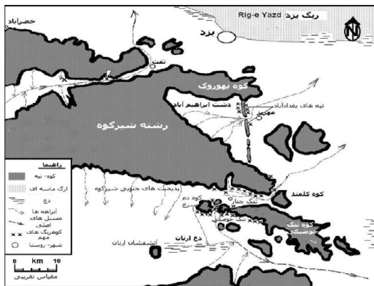
شکل ۵: موقعیت کوهریگ های منطقه شبرکوه یزد در مجاورت ارتفاعات مأخذ: نگارنده
