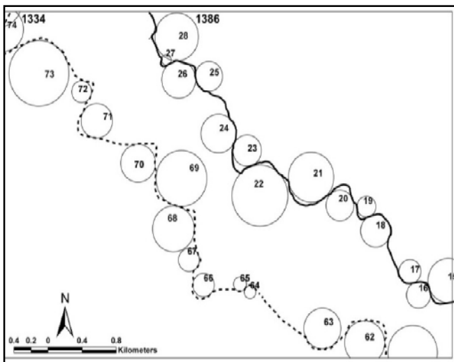
شکل ۳: تغییرات مورفولوژی رودخانه هررود از سال ۱۳۳۴ تا ۱۳۸۶ در قسمت پایانی بازه اول مأخذ: نگارندگان
