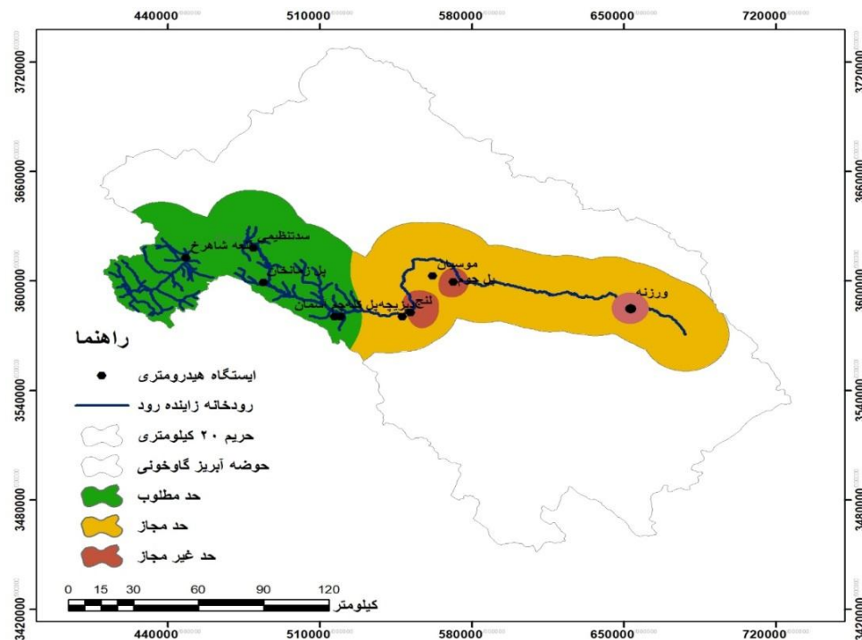
شکل ۳: طبقه‌بندی عناصر کیفی آب زاینده‌رود (۱۳۸۵)
