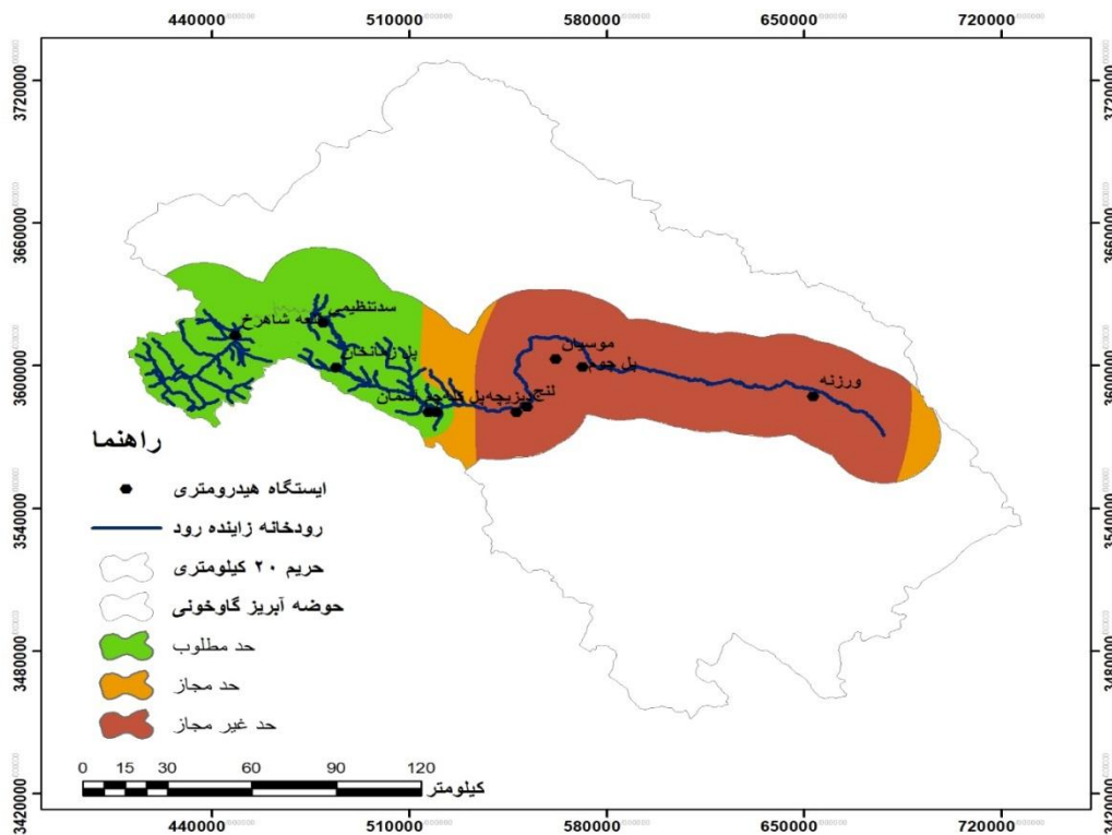
شکل ۶: طبقه‌بندی کیفیت آب زاینده‌رود (۱۳۹۲)
