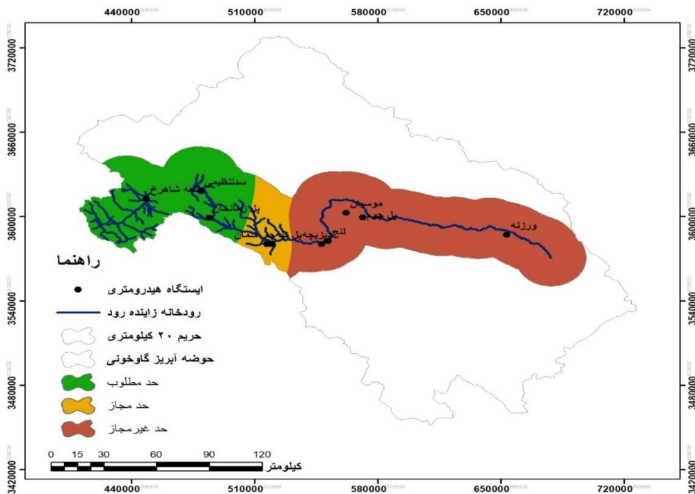
شکل ۷: طبقه‌بندی کیفیت آب زاینده‌رود (۱۳۹۲)
