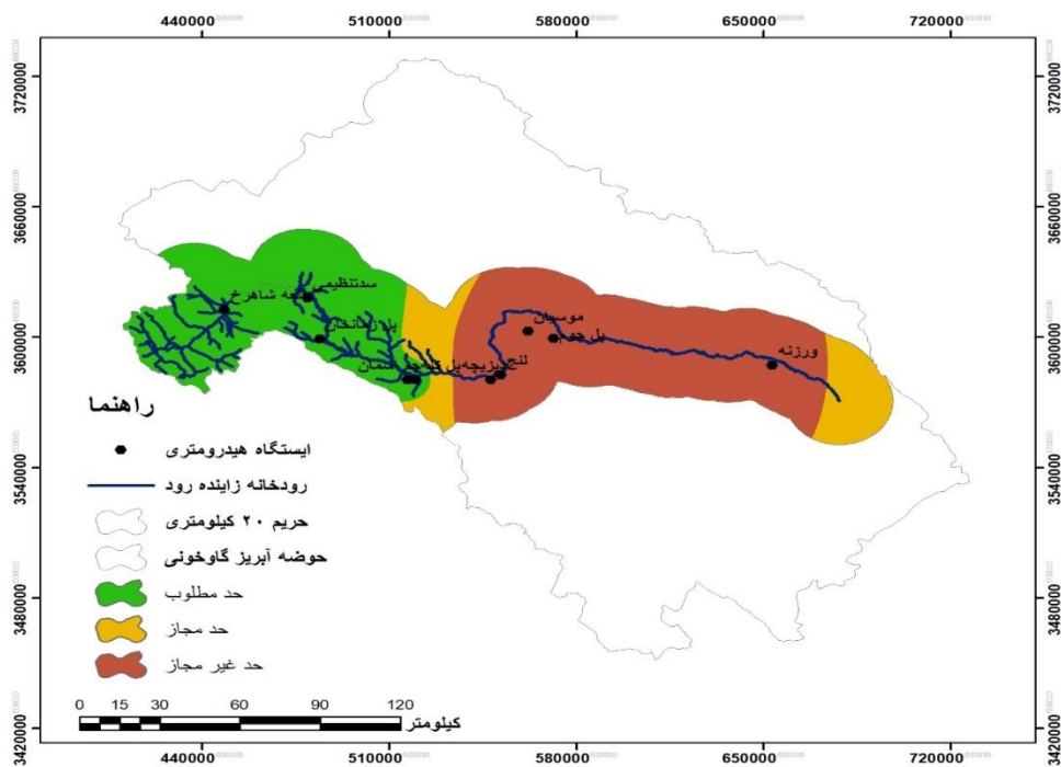
شکل ۵: طبقه‌بندی کیفیت آب زاینده رود (۱۳۹۱)
