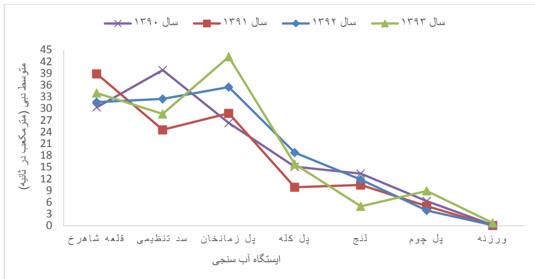
شکل ۲: تغییرات دبی متوسط ایستگاه‌های آب‌سنجی رودخانه زاینده‌رود در سال‌های (۱۳۹۰-۱۳۹۳)
