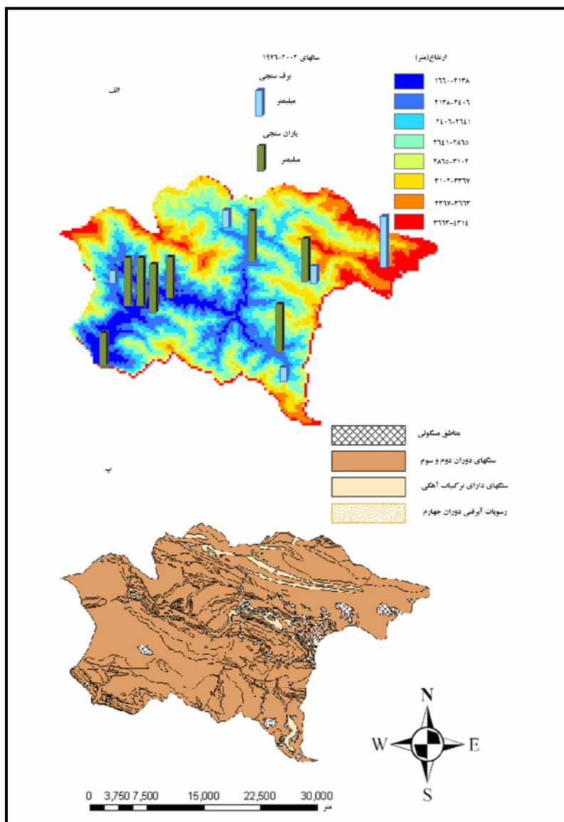
شکل ۲: الف- ایستگاه‌های کلیما تولوژی. ب- نقشه‌ی سنگ شناسی
