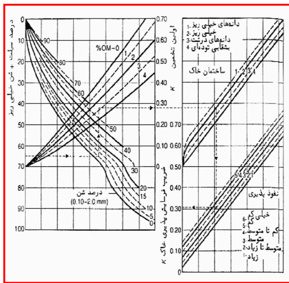
شکل ۲: نمودار فرسایش پذیری خاک تهیه و ترسیم: نگارندگان، ۱۳۹۲
