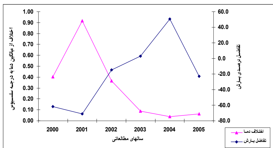
شکل ۳: نوسانات دما و بارش کشور طی سال‌های ۲۰۰۰ تا ۲۰۰۵، نسبت به میانگین درازمدت (۱۹۶۰ تا ۱۹۹۰)
