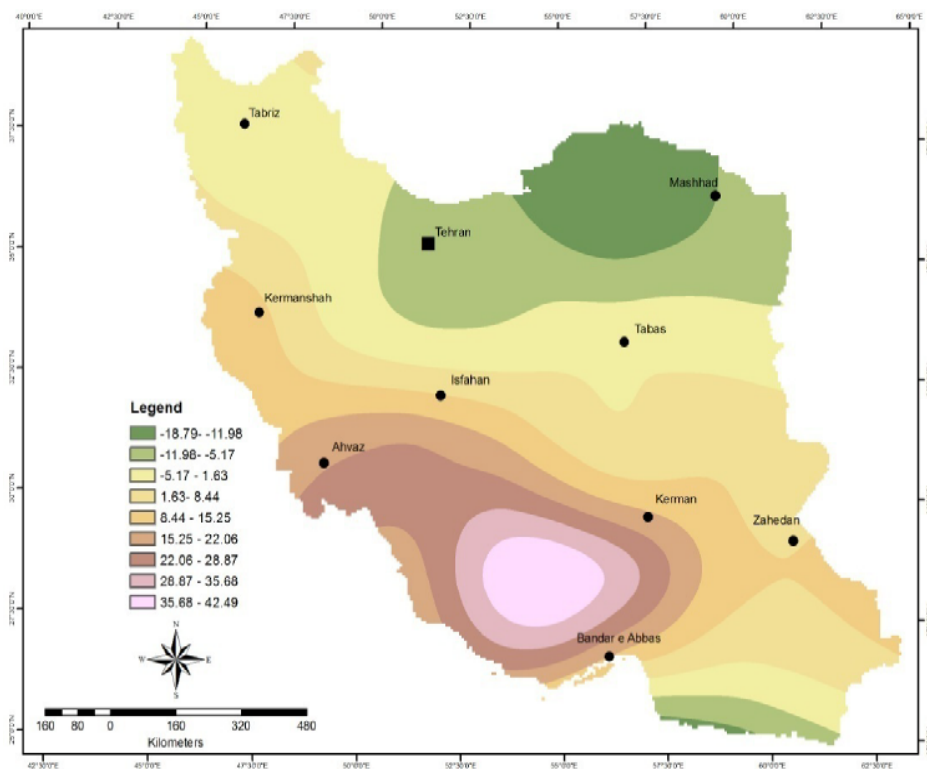
شکل ۱۱: شبیه‌سازی مقادیر بارش با استفاده از نتایج ترکیبی دو مدل GISS—EH و CNRM-CM3 برای سال ۲۰۵۰ مأخذ: نگارندگان
