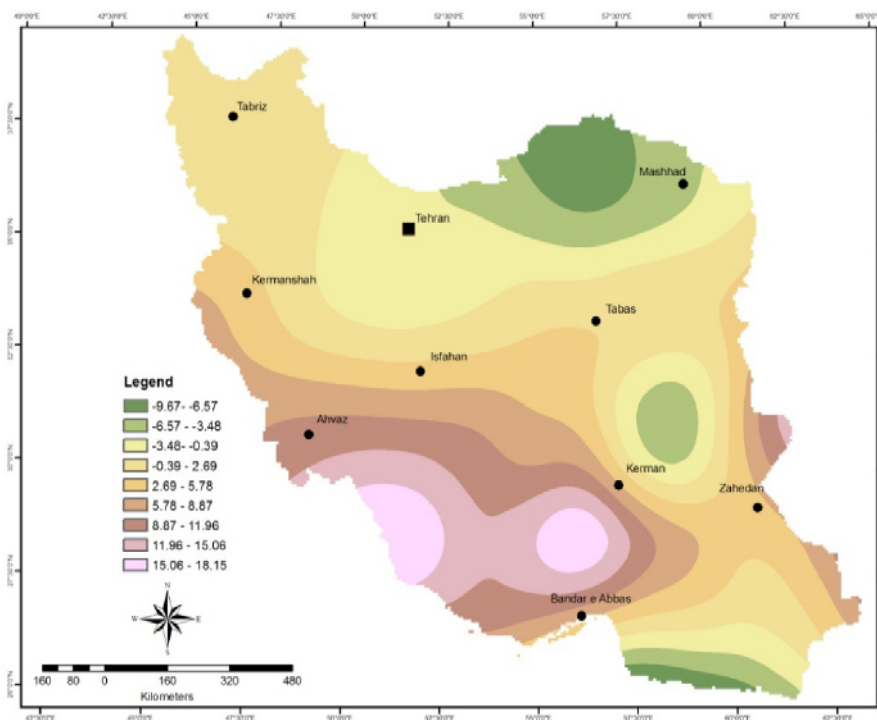
شکل ۱۰: شبیه‌سازی مقادیر بارش با استفاده از نتایج ترکیبی دو مدل GISS—EH و CNRM-CM3 برای سال ۲۰۲۵ مأخذ: نگارندگان
