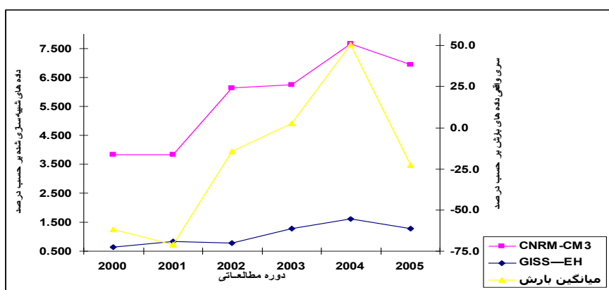
شکل ۷: مقایسه بین سری داده‌های شبیه‌سازی شده بارش توسط دو مدل GISS-EH و CNRM-CM3 با سری واقعی بارش در دوره‌ی مطالعاتی (۲۰۰۵-۲۰۰۰)
