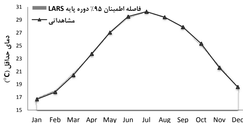
شکل ۲: مقایسه‌ی میانگین بوت استرپی دمای حداقل مشاهداتی در ۹۵٪ فاصله اطمینان داده‌های مدل در ایستگاه سینوپتیک جاسک مأخذ: مطالعات میدانی نگارندگان، ۱۳۹۱
