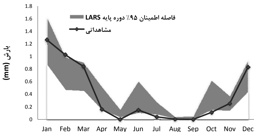
شکل ۴: مقایسه‌ی میانگین بوت استرپی بارش مشاهداتی در ۹۵٪ فاصله اطمینان داده‌های مدل در ایستگاه سینوپتیک جاسک مأخذ: مطالعات میدانی نگارندگان، ۱۳۹۱
