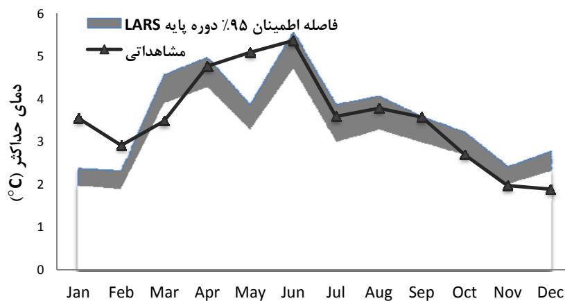
شکل ۶: مقایسه‌ی واریانس بوت استرپی دمای حداکثر مشاهداتی در ۹۵٪ فاصله اطمینان داده‌های مدل در ایستگاه سینوپتیک جاسک مأخذ: مطالعات میدانی نگارندگان، ۱۳۹۱
