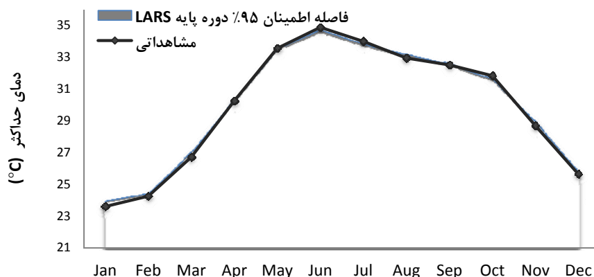
شکل ۳: مقایسه‌ی میانگین بوت استرپی دمای حداکثر مشاهداتی در ۹۵٪ فاصله اطمینان داده‌های مدل در ایستگاه سینوپتیک جاسک مأخذ: مطالعات میدانی نگارندگان، ۱۳۹۱
