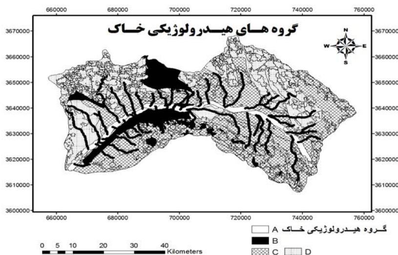
شکل ۷: طبقه‌بندی دشت بیرجند بر اساس گروه‌های هیدرولوژیکی خاک
