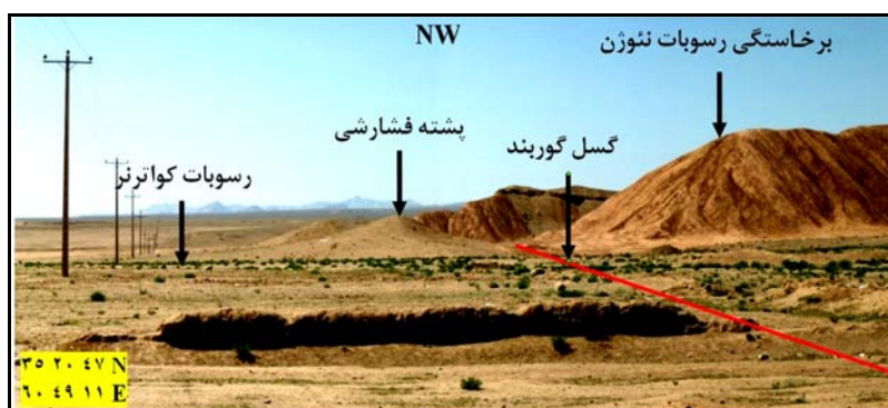
شکل ۱۷: پشته فشارشی ایجاد شده بر اثر عملکرد گسل گوربند
