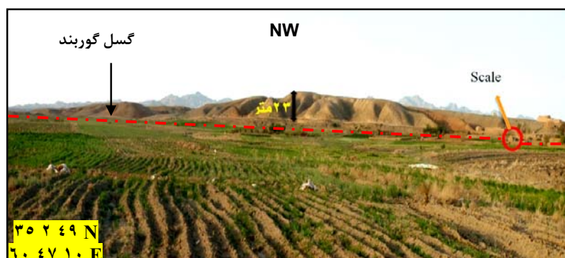
شکل ۱۱: تصویر افزایش گسلی در مجاور روستای گوربند
