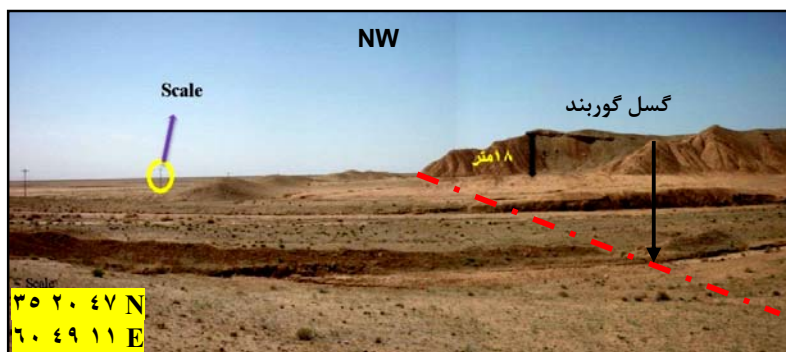
شکل ۹: افزایش گسلی سطح افراز در تصویر دیده می‌شود مأخذ: جامی، ۱۳۹۰
