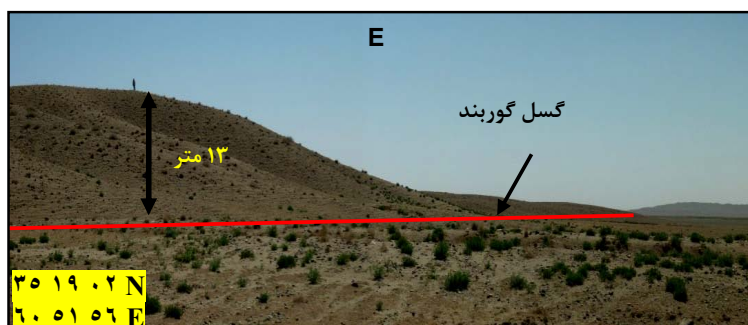
شکل ۱۲: تصویر افزایش گسلی در مجاور روستای قلعه گک
