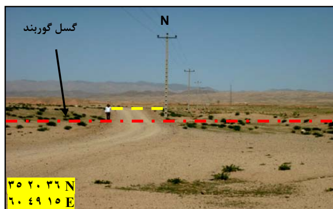
شکل ۱۰: فرازش زمین در محل اثر سطحی گسل گوربند در رسوبات کواترنر مأخذ: جامی، ۱۳۹۰
