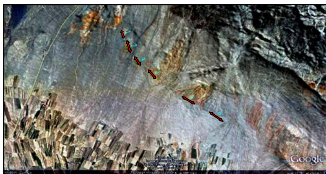
شکل ۶: تصویر موقعیت مقاطع انتخابی برای تعیین سینوسیتی پیشانی کوهستان
