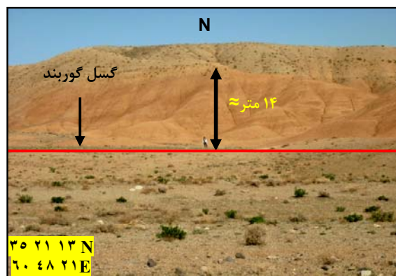
شکل ۸: افزایش گسلی در محل اثر سطحی گسل در رسوبات کواترنر مأخذ: جامی، ۱۳۹۰
