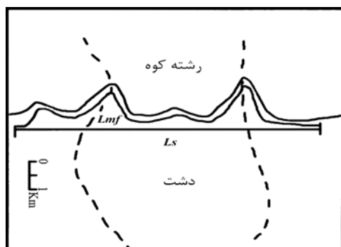
شکل ۵: نحوه محاسبه شاخص Smf مأخذ: پورکرمانی و سلگی، ۱۳۸۸
