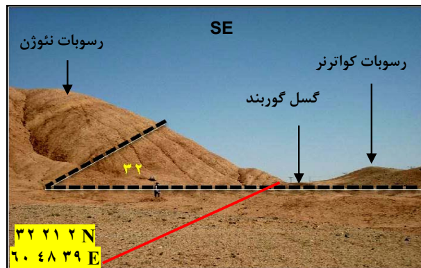
شکل ۱۹: زاویه شیب لایه‌ها در منطقه گسلی مجاور روستای تغز
