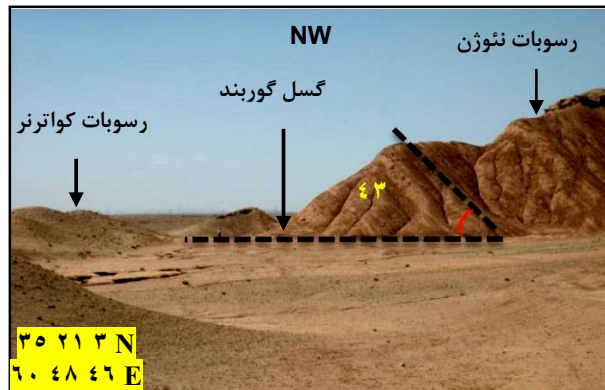
شکل ۱۸: زاویه شیب لایه‌ها در منطقه گسلی مجاور روستای گوربند
