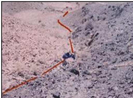
شکل ۱۴: کنتاکت (خط تیره) بین سنگ‌های رسوبی (قسمت روشن) با سنگ‌های آذرینی (قسمت تیره) و وجود گسل موقعیت: 31^{\circ} 38' 15'' N 60^{\circ} 12' 47'' E جهت دید عکس: جنوب غرب
