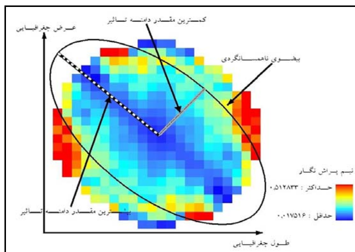
شکل ۲: رویه‌ی پراش نگار و بیضوی ناهمسانگردی
