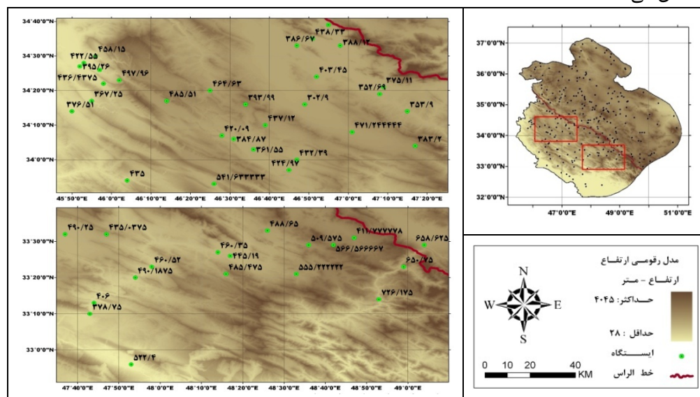
شکل ۷: اثر تخلیه‌ی رطوبتی توده‌های هوا با رسیدن به خط‌الرأس‌ها، مناطق مشخص شده (کادر قرمز رنگ) به ترتیب بزرگنمایی شده و در سمت چپ نمایش داده شده‌اند.
