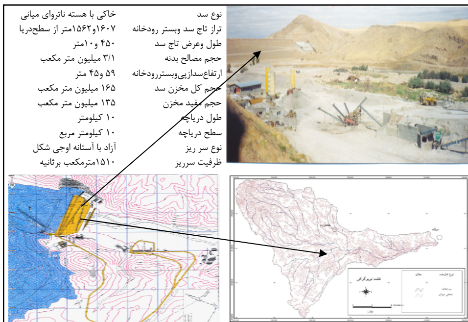
شکل ۳: مشخصات، محل و عملیات احداث سد سهند و مواد انباشته شده در بستر ناشی از عملیات اجرایی
