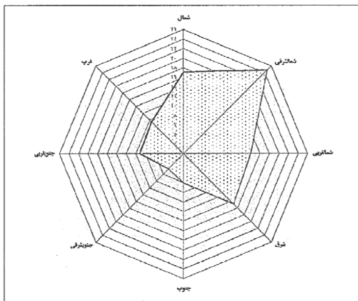
شکل ۱۲: نمودار کلاس بندی شیب در حوضه در پرچین
