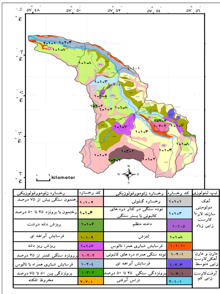
شکل ۷: نقشه ژئومورفولوژی حوضه درپچین
