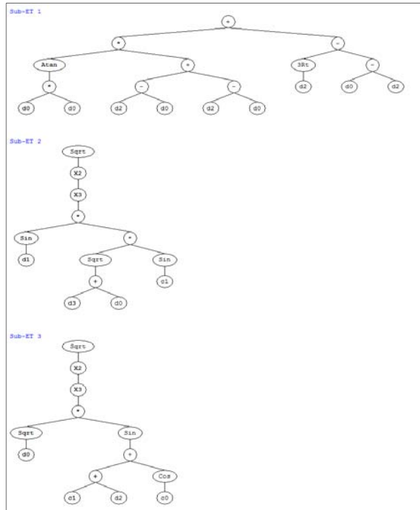
شکل ۱۰: بیان درختی زن‌های ۱، ۲ و ۳ در سناریوی دوم پیش‌بینی بار رسوب معلق ایستگاه هیدرومتری پای پل
