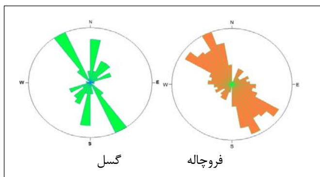
شکل ۷: نمودار گلسرخه کشیدگی محور اصلی فروچاله‌ها و گسل‌ها مأخذ: مطالعات میدانی نگارندگان، ۱۳۹۱
