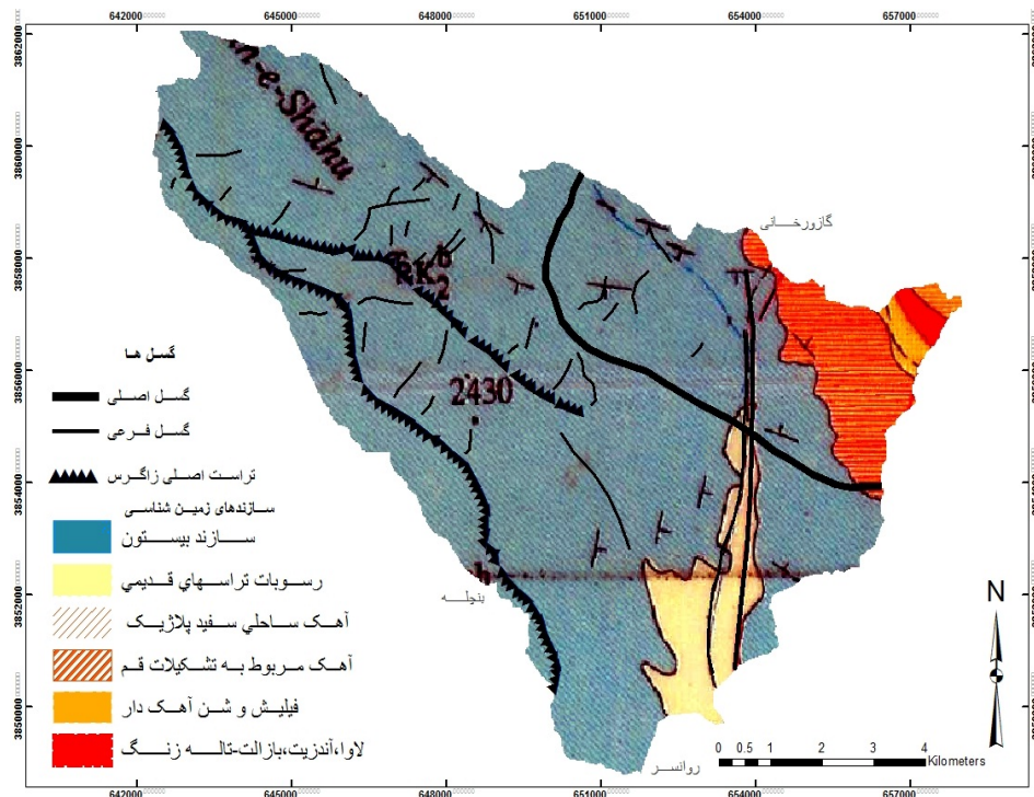
شکل ۲: نقشه زمین‌شناسی و گسل‌های منطقه
