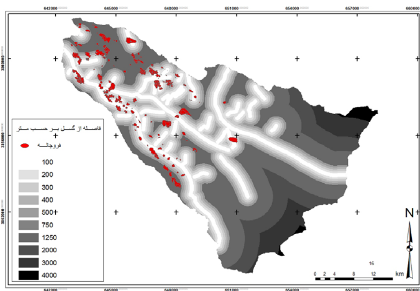
شکل ۸: فروچاله‌ها در ارتباط با میزان فاصله از گسل مأخذ: مطالعات میدانی نگارندگان، ۱۳۹۱
