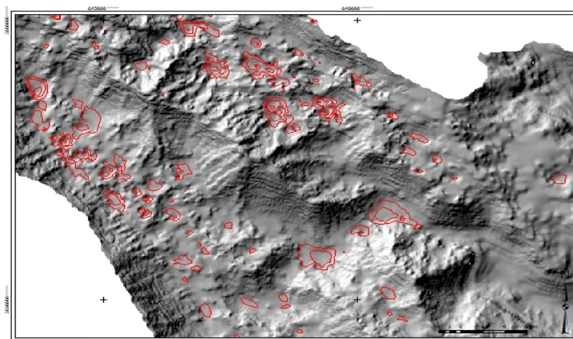
شکل ۴: انواع فروچاله‌ها در منطقه گازورخانی بر اساس مورفولوژی - برگرفته از ۱۰dem متر منطقه
