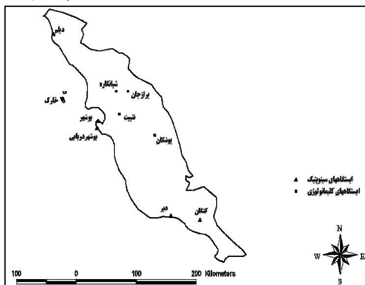
شکل ۲۳: موقعیت ایستگاههای سینوپتیک و کلیماتولوژی استان بوشهر
