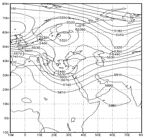
شکل ۲۲: الگوی آرایش پربندی در تراز ۵۰۰ هکتوپاسکال روز ۱۳۸۲/۱۰/۲۰
