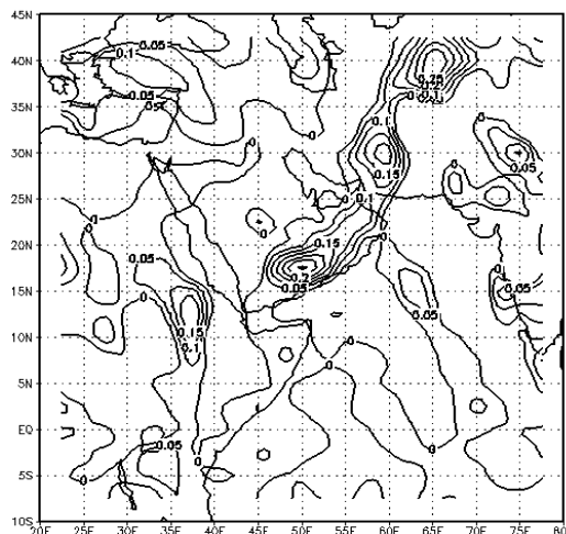
شکل ۳: نقشه‌ی وزش رطوبتی تراز دریا روز ۱۳۸۲/۰۹/۱۶
