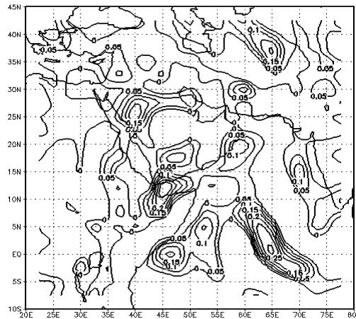
شکل ۲۱: نقشه‌ی وزش رطوبتی تراز ۸۵۰ هکتوپاسکال روز ۱۳۸۲/۱۰/۲۰
