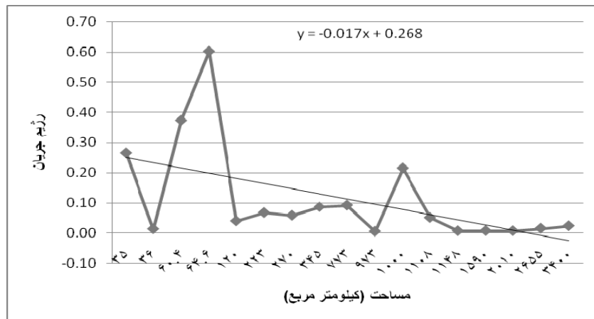
شکل ۱۲: رابطه‌ی مساحت و رژیم رسوب در دوره‌ی بازگشت ۲ سال مأخذ: مطالعات میدانی نگارندگان، ۱۳۹۰
