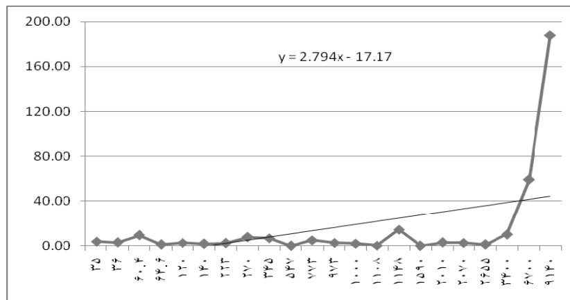
شکل ۱۳: رابطه‌ی مساحت و رژیم رسوب در دوره‌ی بازگشت ۱۰۰ سال مأخذ: مطالعات میدانی نگارندگان، ۱۳۹۰
