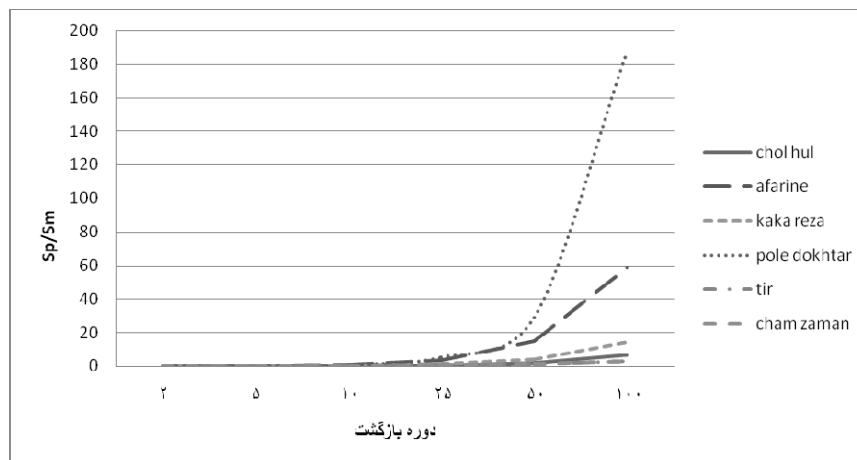
شکل ۷: مقادیر رژیم رسوب با دوره‌ی بازگشت‌های مختلف در ایستگاه‌های منتخب (Sp عبارت است از میزان رسوب
