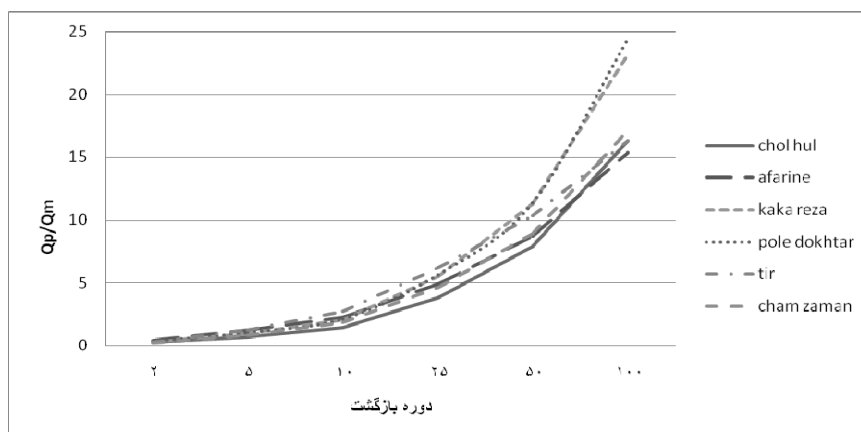
شکل ۴: وضعیت رژیم جریان با دوره‌ی بازگشت‌های مختلف در ۶ ایستگاه منتخب (Qp دبی پیک با دوره بازگشت‌های مختلف است و Qm دبی میانگین می‌باشد) مأخذ: مطالعات میدانی نگارندگان، ۱۳۹۰
