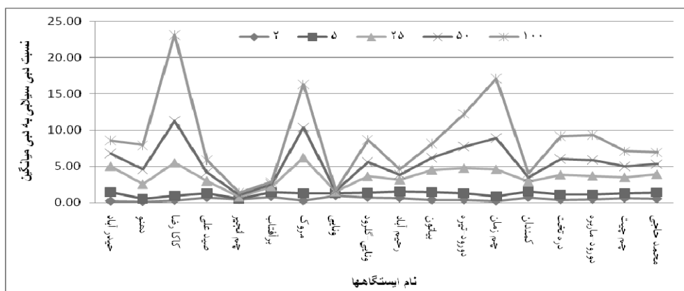
شکل ۳: وضعیت رژیم جریان با دوره بازگشت‌های مختلف در هر ایستگاه مأخذ: مطالعات میدانی نگارندگان، ۱۳۹۰
