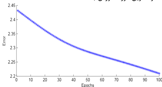
شکل ۱۶: کاهش میزان خطای آموزش مدل با افزایش تعداد تکرار مأخذ: مطالعات میدانی نگارندگان، ۱۳۹۱
