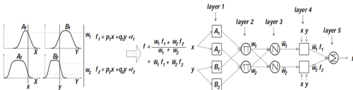
شکل ۱: یک سیستم فازی سوگنو با تابع عضویت فوسی و سیستم ANFIS معادل با آن مأخذ: Jang, 1993
