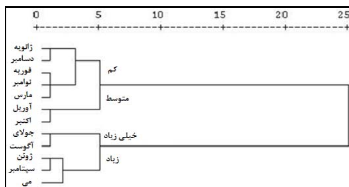
شکل ۳: دندروگرام ماهانه گرد و غبار در ایستگاه سینوپتیک زابل
