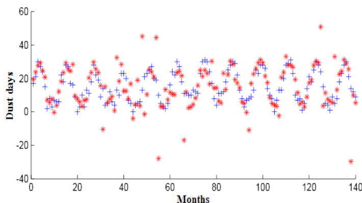
شکل ۱۷: مقایسه داده پیش بینی شده و اعتبارسنجی گرد و غبار در ایستگاه زابل
