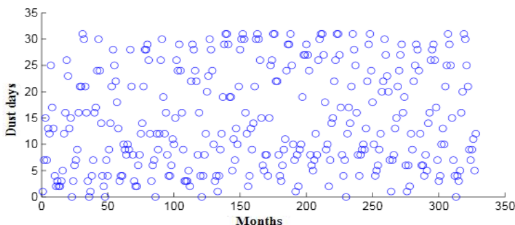
شکل ۱۱: داده‌های آموزشی تعیین شده گرد و غبار
