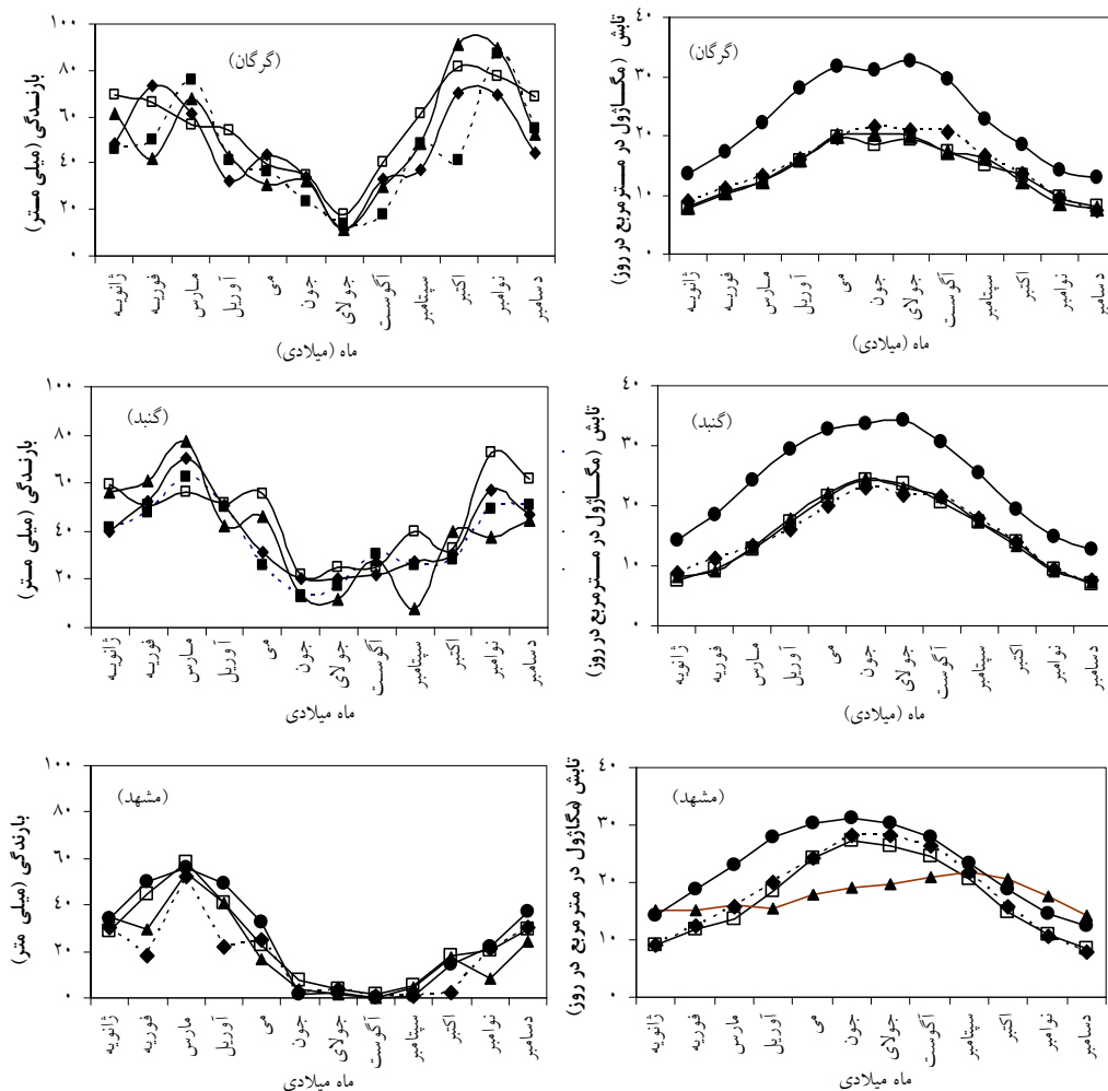
شکل ۲: مقایسه‌ی میانگین ماهانه ۱۰ ساله داده‌های مشاهده شده (♦♦♦♦) و شبیه‌سازی شده با مدل‌های CLIMGEN (—▲—) و LARS (—●—) WeatherMan و WG (—□—) برای پارامترهای تابش و بارندگی سال‌های ۲۰۰۹-۲۰۰۰ در اقلیم‌های گرجان، گنبد و مشهد مأخذ: مطالعات میدانی نگارندگان، ۱۳۹۰: ۲۳
