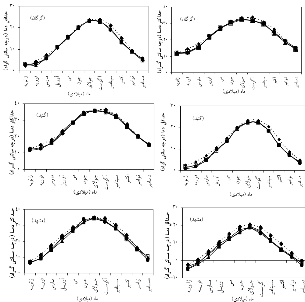
شکل ۱: مقایسه‌ی میانگین ماهانه ۱۰ ساله داده‌های مشاهده شده (---◆---) و شبیه‌سازی شده با مدل‌های CLIMGEN (---●---) WeatherMan و (—■—) LARS-WG، برای حداقل و حداکثر دمای سال‌های ۲۰۰۹-۲۰۰۰
