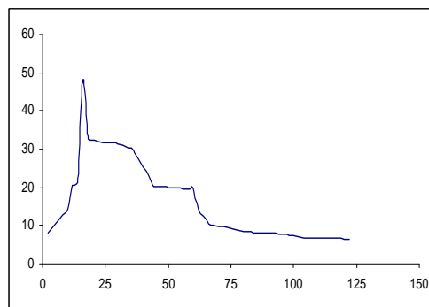
شکل ۲: هیدروگراف سیل ۱۳۶۶/۱۱/۲۵
