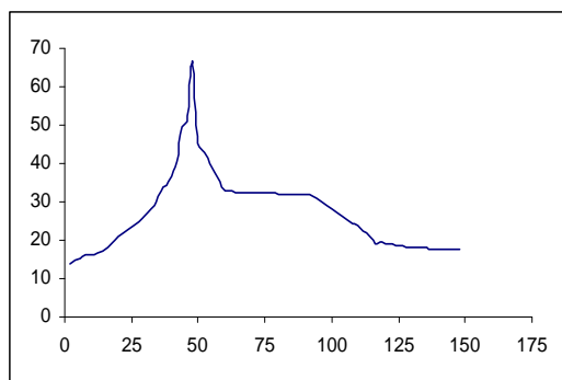
شکل ۳: هیدروگراف سیل ۱۳۶۶/۸/۰۳
