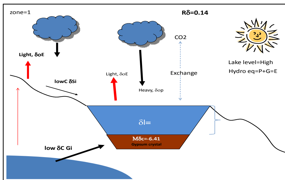
شکل ۶: (\delta O^E) مقادیر ایزوتوپ اکسیژن تبخیر (\delta C^{Si}) مقادیر ایزوتوپ کربن آب‌های سطحی (\delta C^{Gi}) مقادیر ایزوتوپ کربن آب‌های زیرزمینی (\delta O^P) مقادیر ایزوتوپ آب باران مأخذ: نگارندگان
