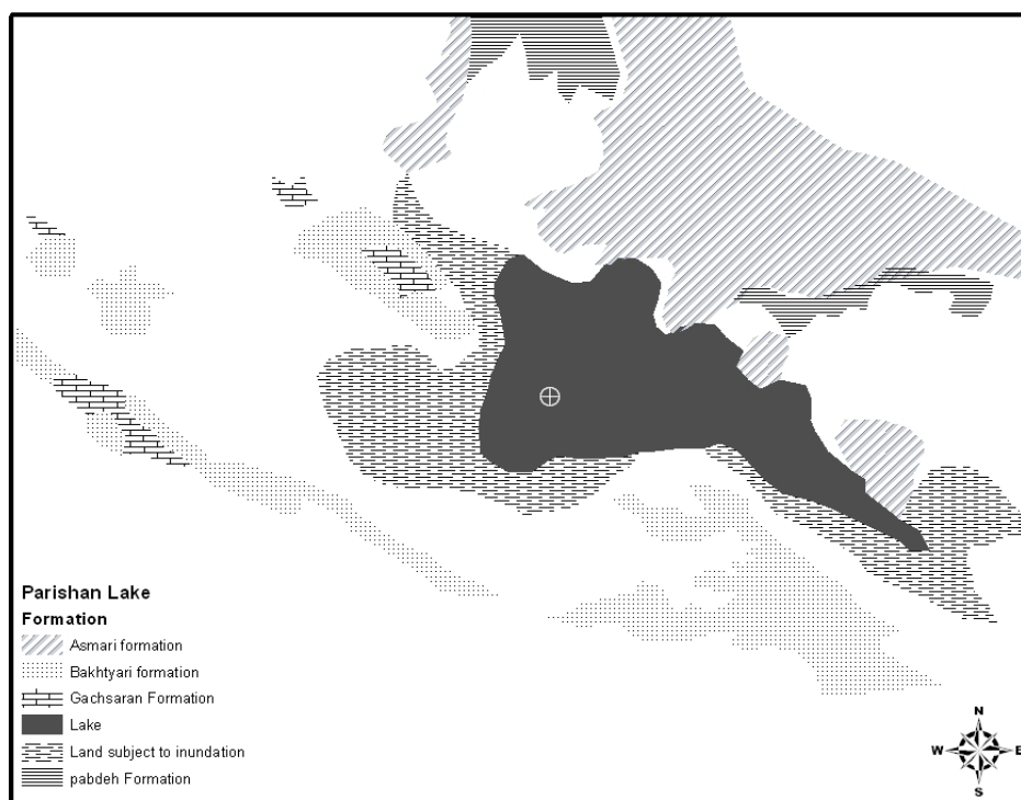
شکل ۱: نقشه بالا: موقعیت دریاچه پریشان نسبت به اسناد مهم دریاچه‌های ارومیه و زریوار در شرق نزدیک نقشه پایین: سازندهای اصلی حاشیه‌ی دریاچه پریشان و موقعیت نقطه برداشت شده
