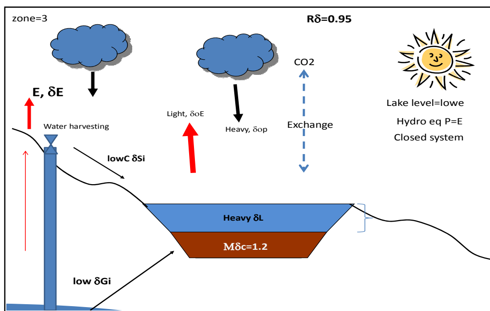
شکل ۸: مقادیر ایزوتوپ اکسیژن تبخیر (δCSi) مقادیر ایزوتوپ کربن آبهای سطحی (δCGi)
