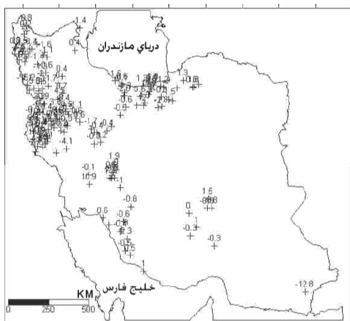
نقشه ۶: انحراف مقادیر برآزش یافته براساس مدل نمایی نیمه تغییرنا برای ۲۵ درصد ایستگاه های مورد بررسی
