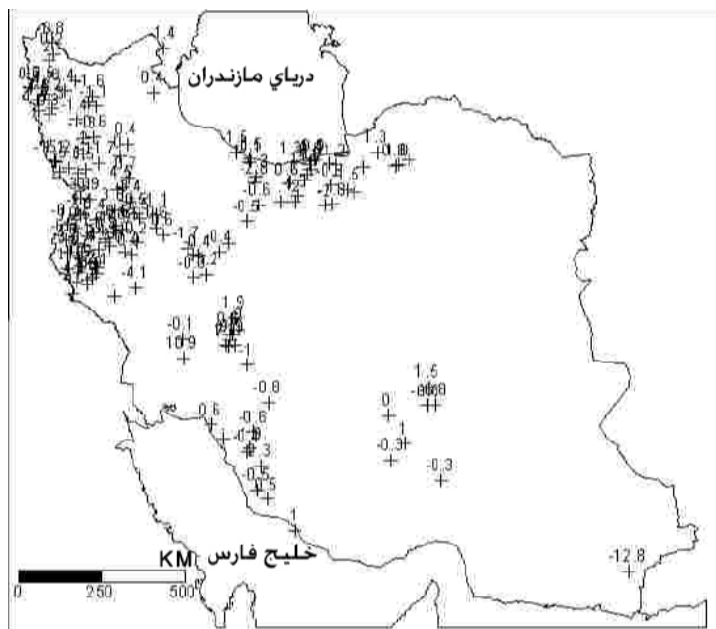
نقشه ۵: انحراف مقادیر برآزش یافته براساس مدل خطی نیمه تغییرنا برای ۲۵ درصد ایستگاه های مورد بررسی
